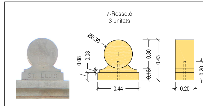
DETALL ROSETÓ
