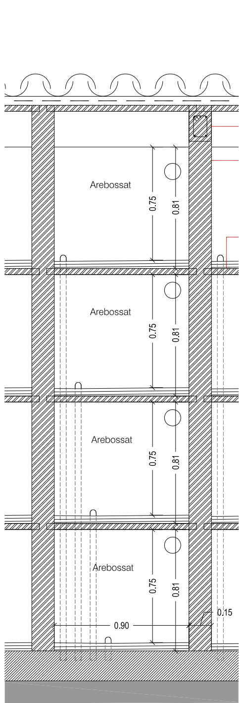
SECCIÓ TRANSVERSAL
