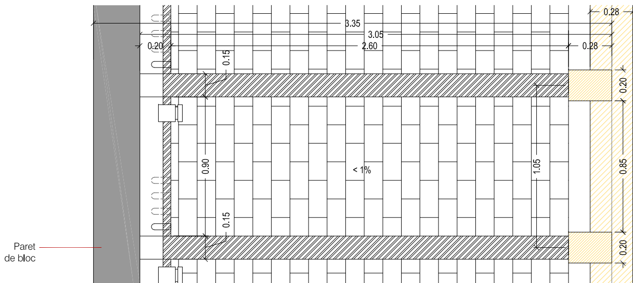
PLANTA
