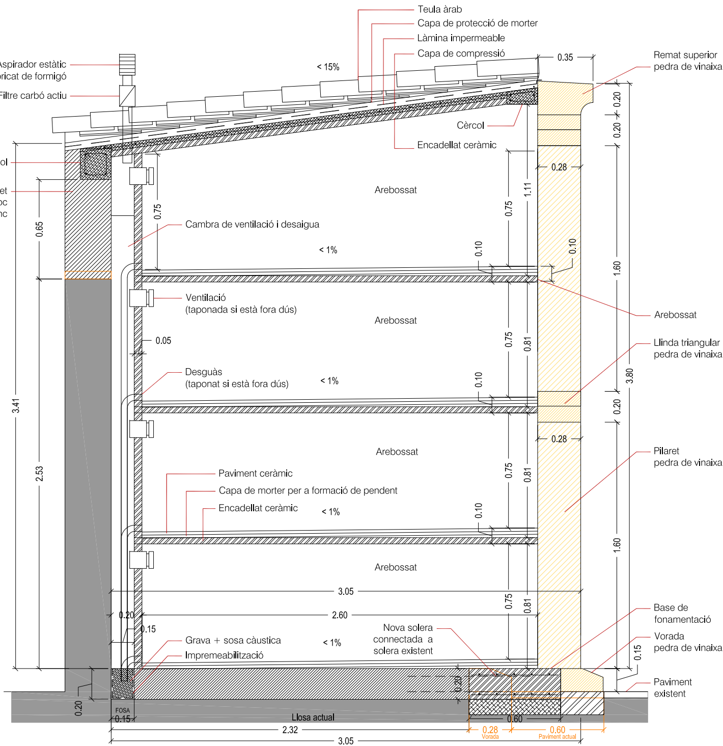
SECCIÓ LONGITUDINAL
